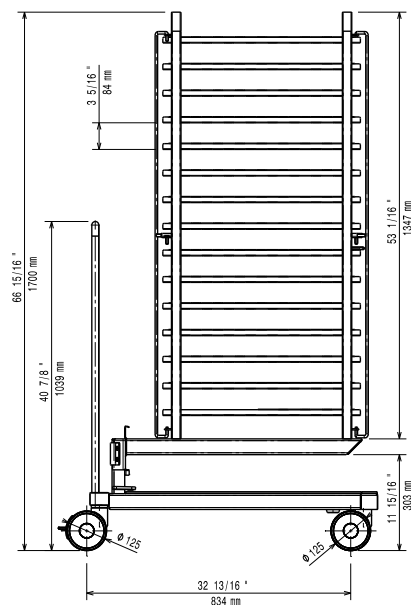
Front aanzicht
