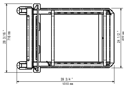
Boven aanzicht
